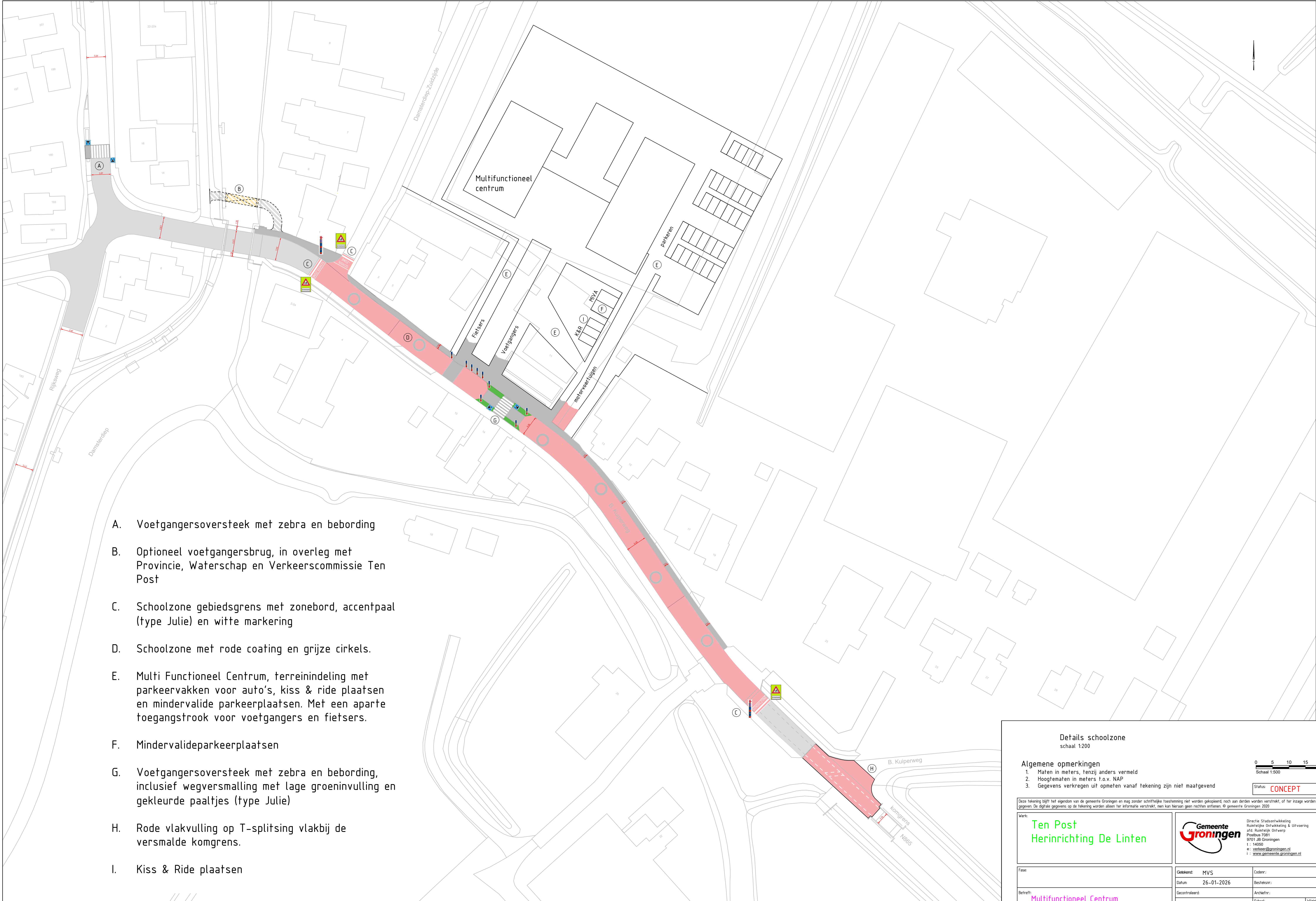
SITUATIE B. KUIPERWEG MET SCHOOLZONE schaal 1:500
